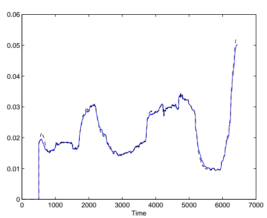
(d) \text{vol}(JPM)(t) (—) and 20 days forecasting (---)
