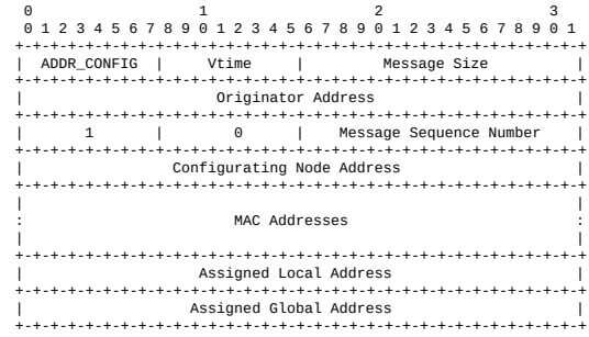
Fig. 4. ADDR_CONFIG message format.
