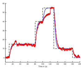
(d) Output variable and reference trajectory
