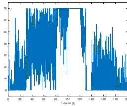
(d) PI: control variable
