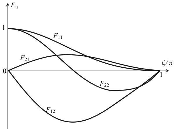
Fig. 1 The F_{ij} 's computed
