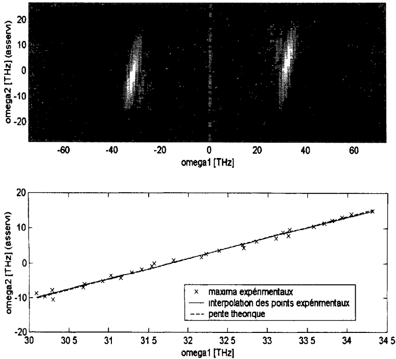
Figure 2. En haut - Double transformée de Fourier de S(\tau, \tau) émis par un cristal d'AgGaS 2 (type I, \phi = \theta = 45^\circ ) épais de 500 \mu\text{m} . En bas - Comparaison des maxima expérimentaux à la courbe d'accord de phase théorique (écart < 2.6%). Le repliement de la carte suivant \omega_2 (variable conjuguée de \tau ) est dû à l'échantillonnage temporel choisi.
