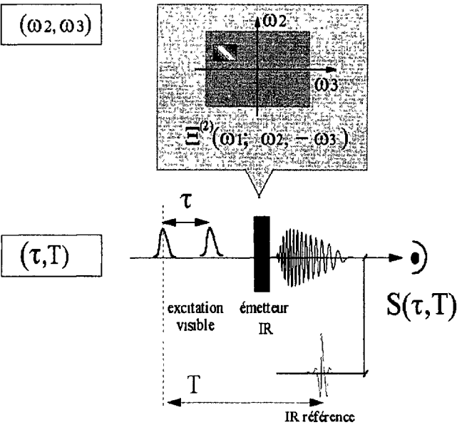
Figure 1. Principe de la spectroscopie non-linéaire à deux dimensions spectrales (ici, dans le cas d'une émission d'infrarouge IR par différence de fréquence \omega_{\text{émission}} = \omega_1 = \omega_3 - \omega_2 )
